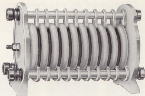
Abbildung 6 Hescho-Kondensatorblock in Serienschaltung (S-Block)
