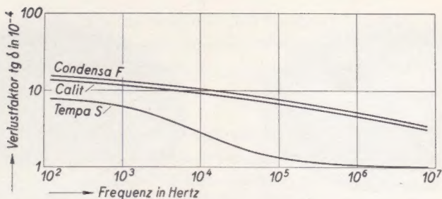
Abbildung 3 Frequenz-Abhängigkeit von \operatorname{tg} \delta bei HF-Kondensatoren aus Calit, Tempa S und Condensa F
