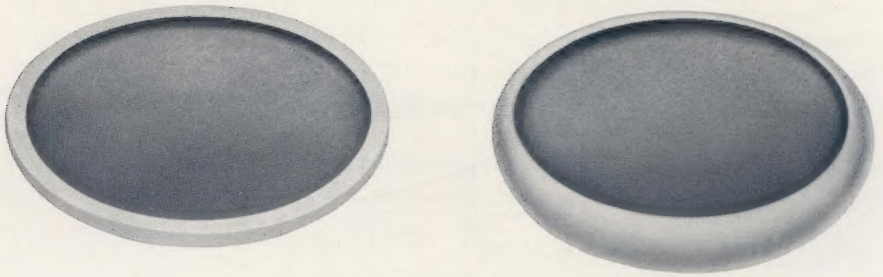
Abbildung 1 Hescho-Plattenkondensatoren (200 mm Dmr.) mit aufgebranntem, metallisch verstärktem Belag und verdicktem oder wulstförmigem Rand als Sprühschutz
